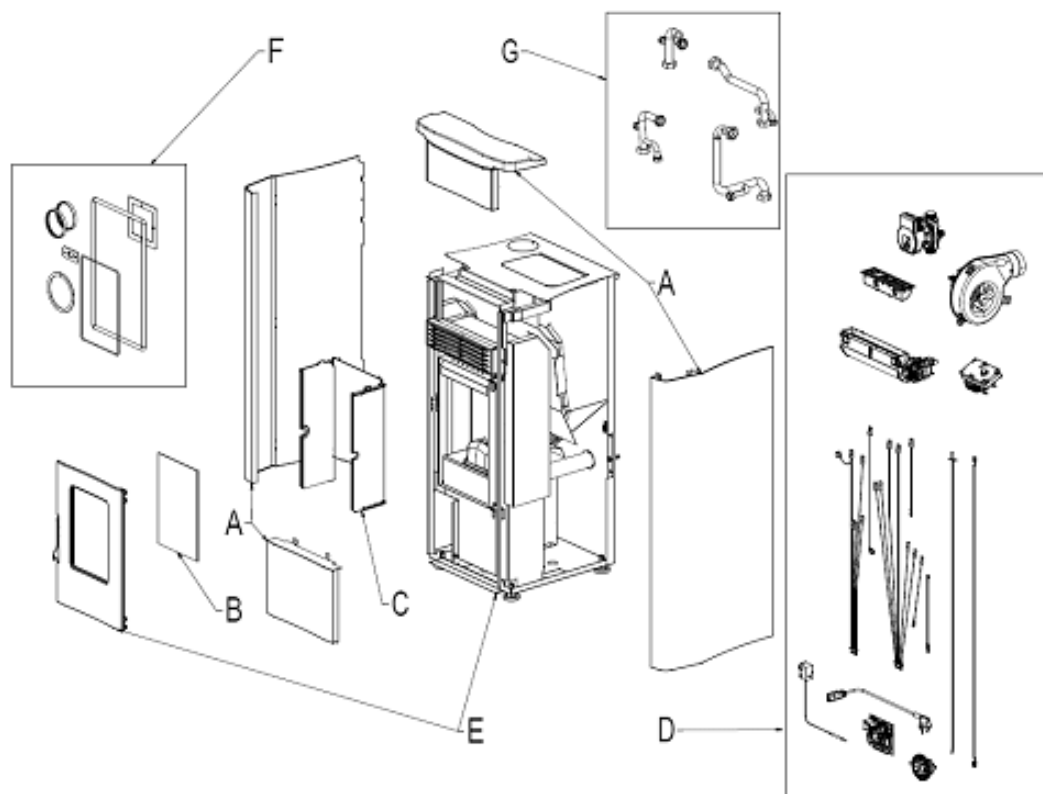
Fig. 1 - Explosionszeichnung
