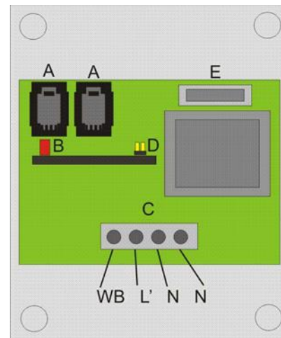
Abbildung 1 Anschlüsse
