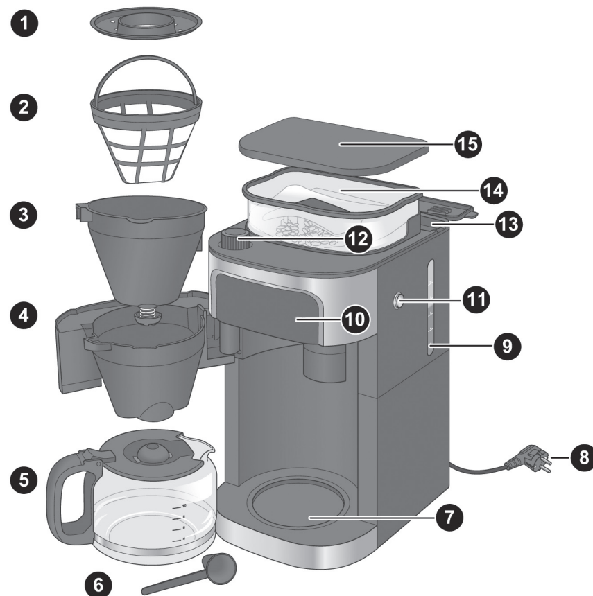
Fig. 1: Partes del aparato
