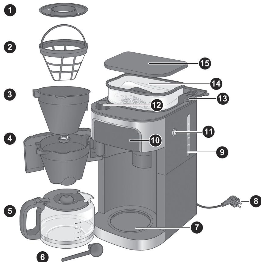
Fig. 1: Partes do aparelho
