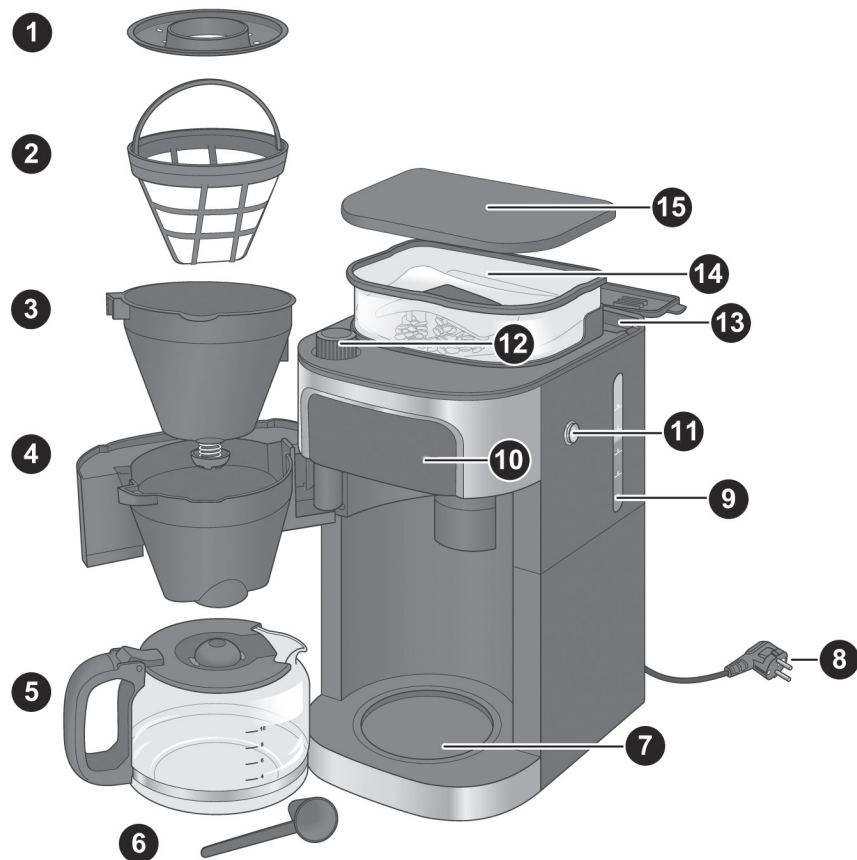
Kuva 1: Laitteen osat
