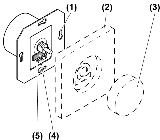
Bild 1: Geräteaufbau
