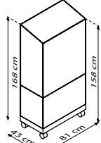
STAD ROLLFUNDAMENT
